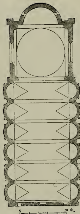
Abb. 152. Carmine zu Padua. (L.)
